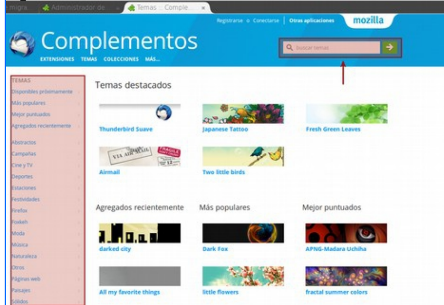
Figura 2: Buscar temas
