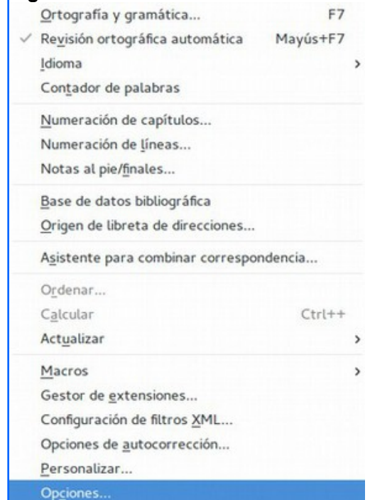
Figura 1: Menú herramientas
